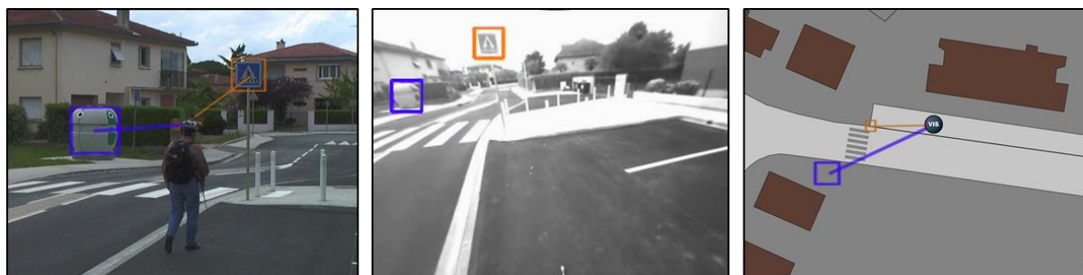
Figure II-22 Positionnement utilisateur basé sur la détection d'amers visuels aux coordonnées connues. Vue extérieure à gauche, image des caméras embarquées au centre droite, et vue de la carte à droite.
